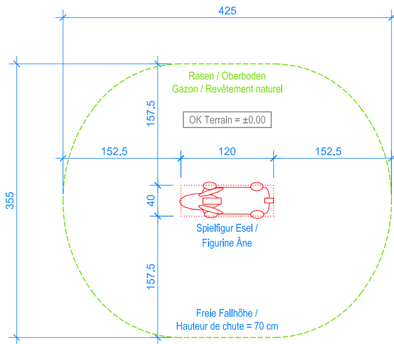
GRUNDRISS / PLAN 1:50
