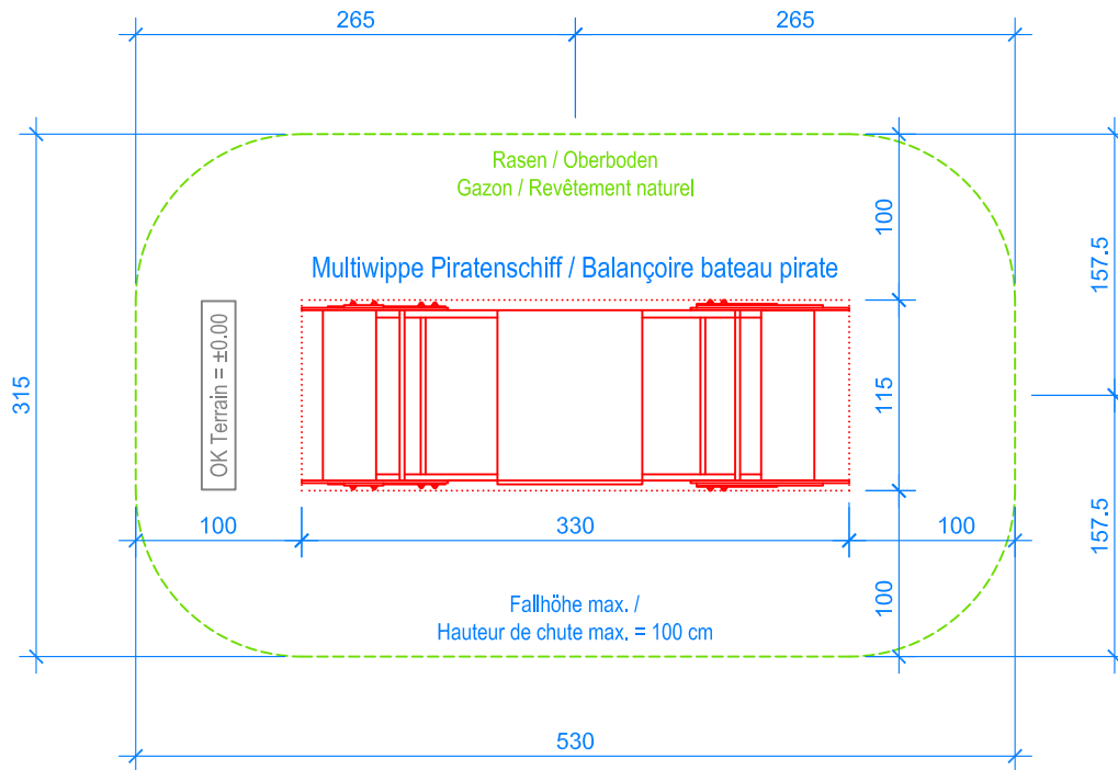
GRUNDRISS / PLAN 1:50
