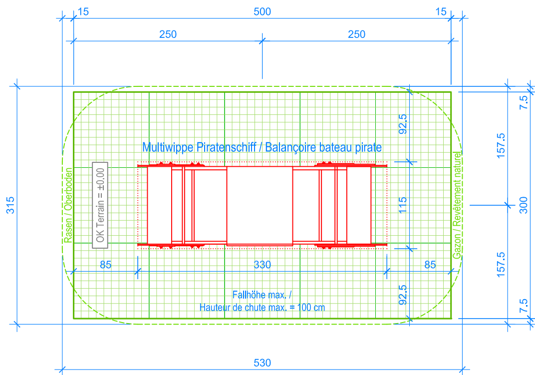
GRUNDRISS / PLAN 1:50
