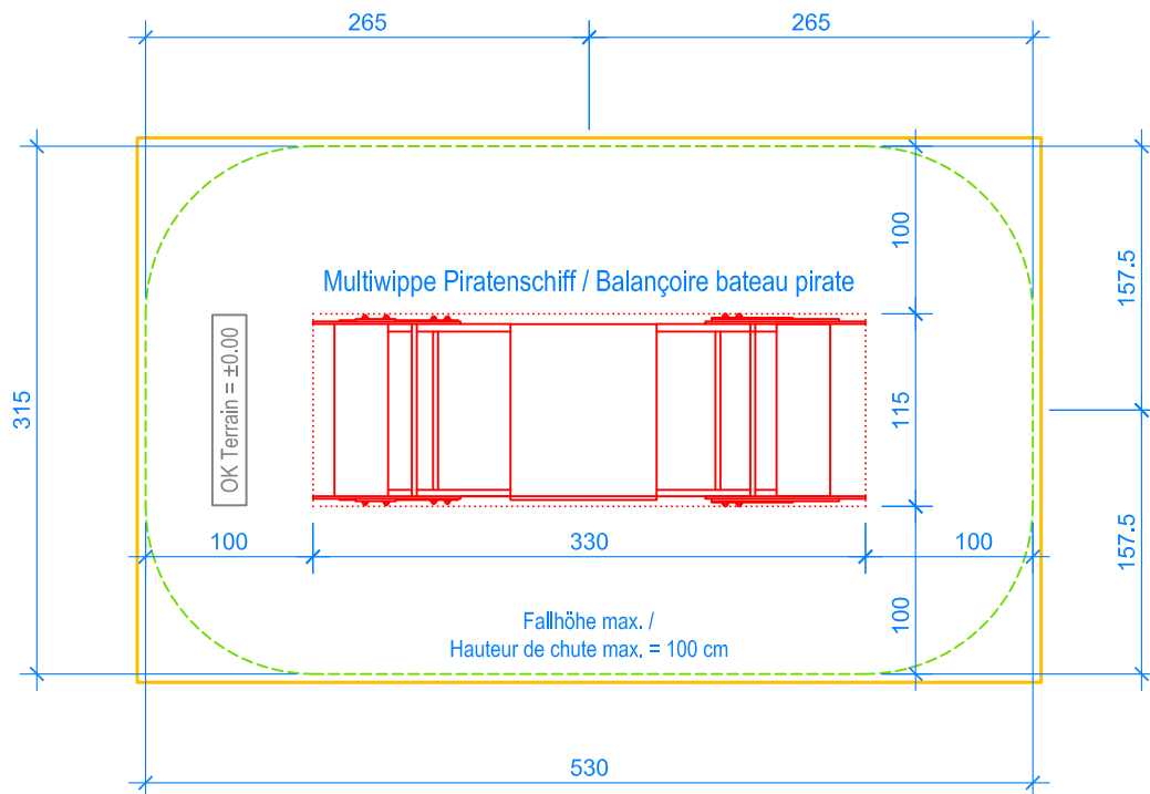
GRUNDRISS / PLAN 1:50
