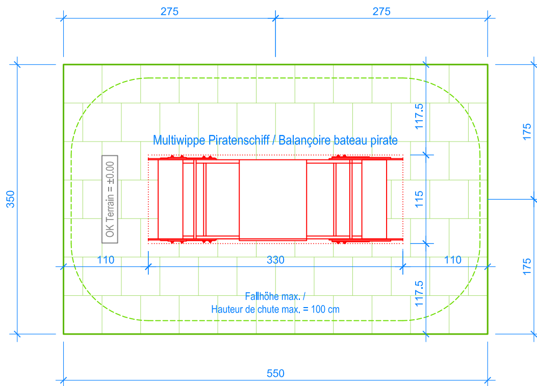
GRUNDRISS / PLAN 1:50
