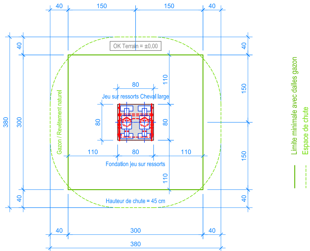
PLAN 1:50
