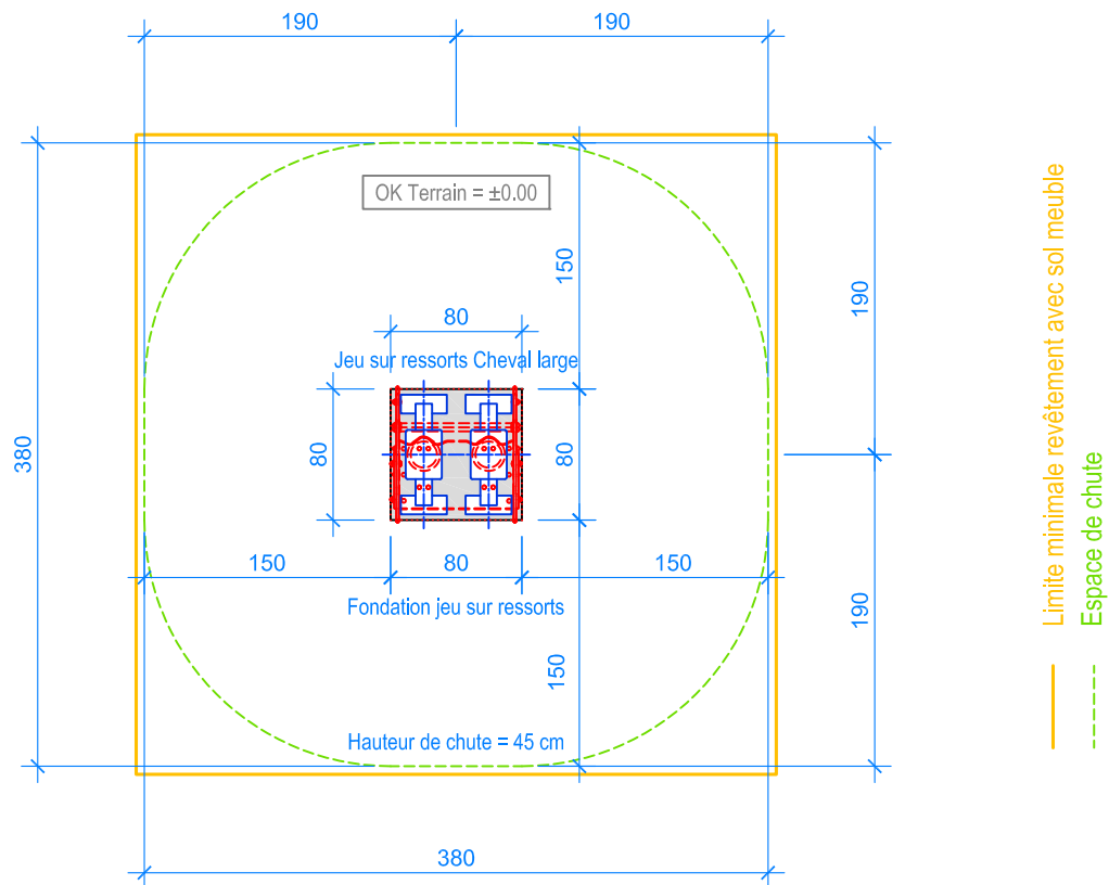
PLAN 1:50
