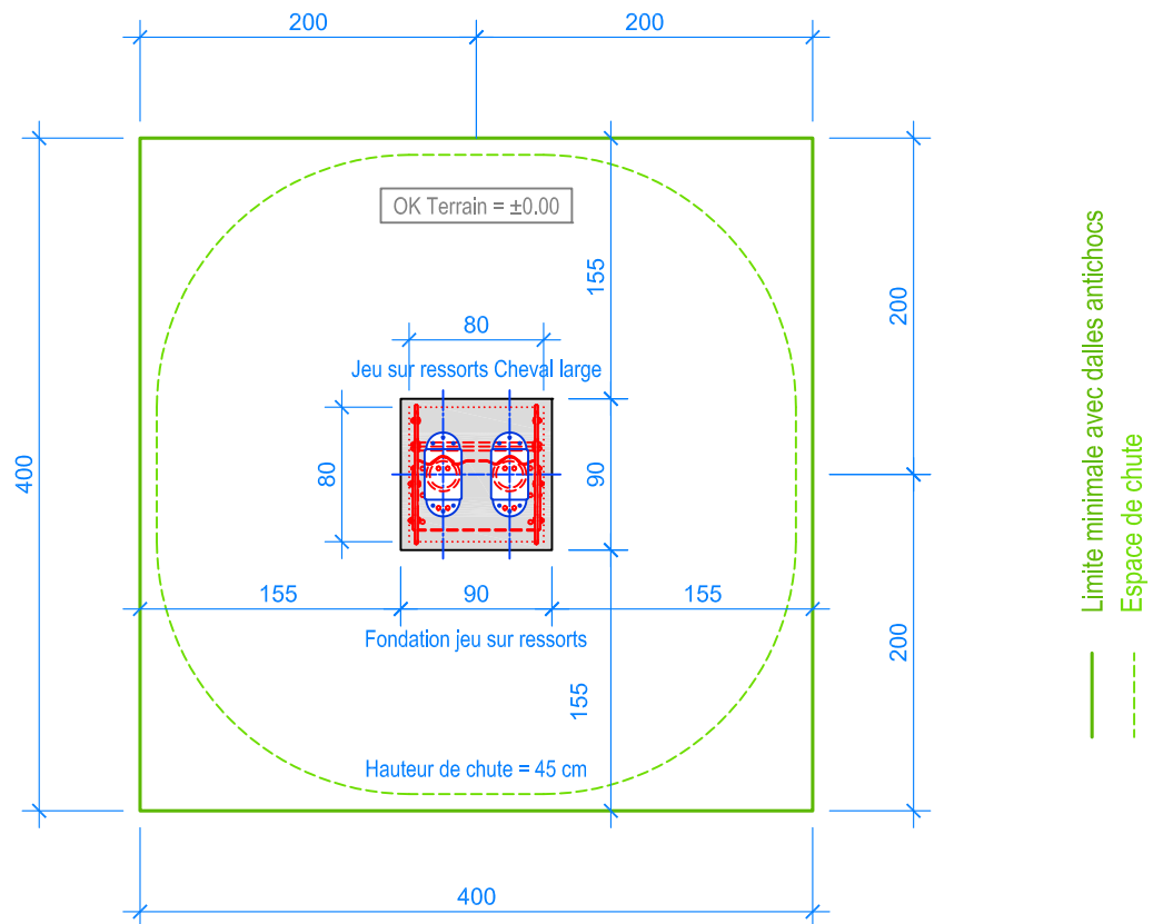
PLAN 1:50
