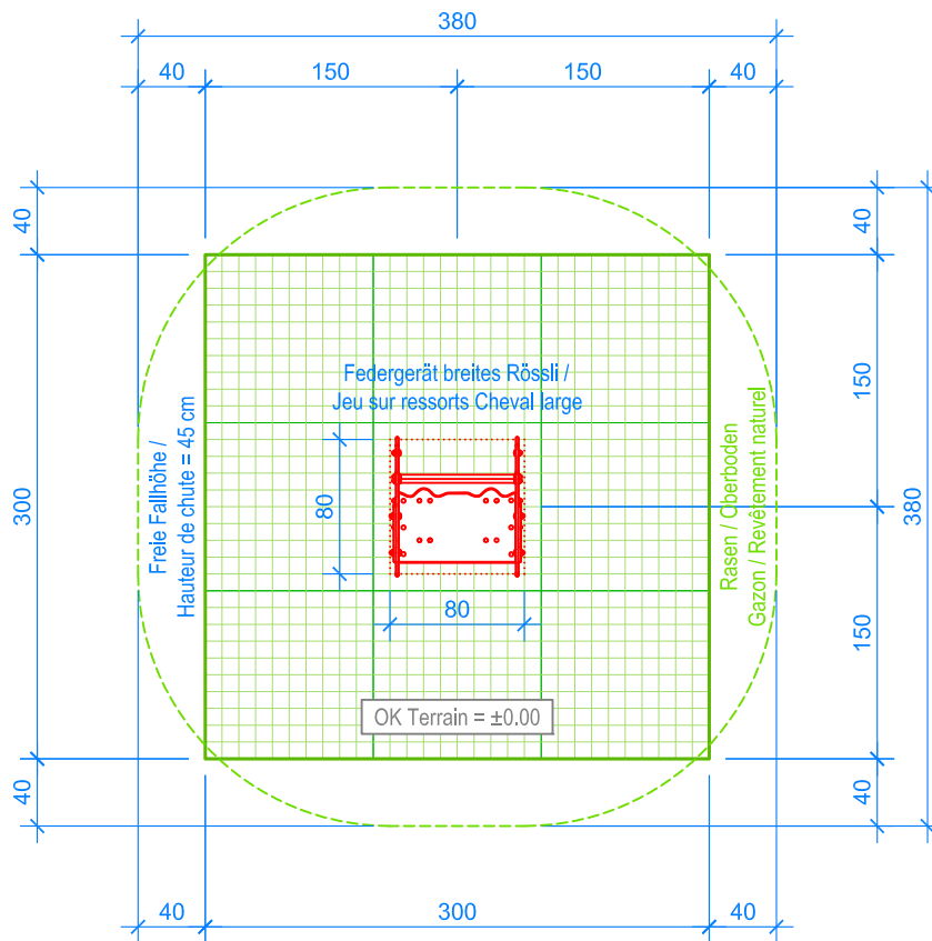
GRUNDRISS / PLAN 1:50
