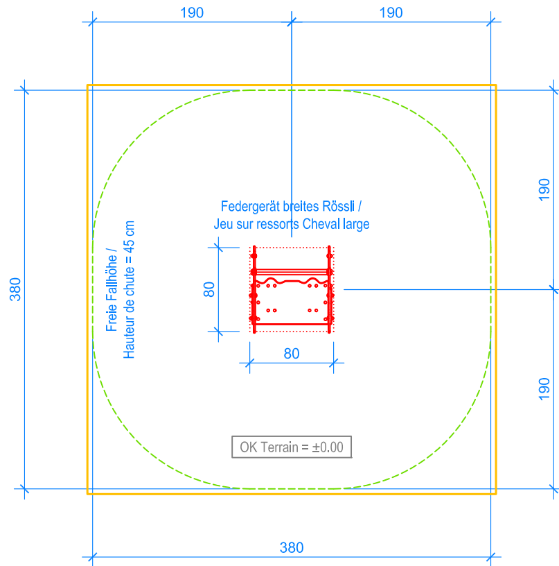
GRUNDRISS / PLAN 1:50
