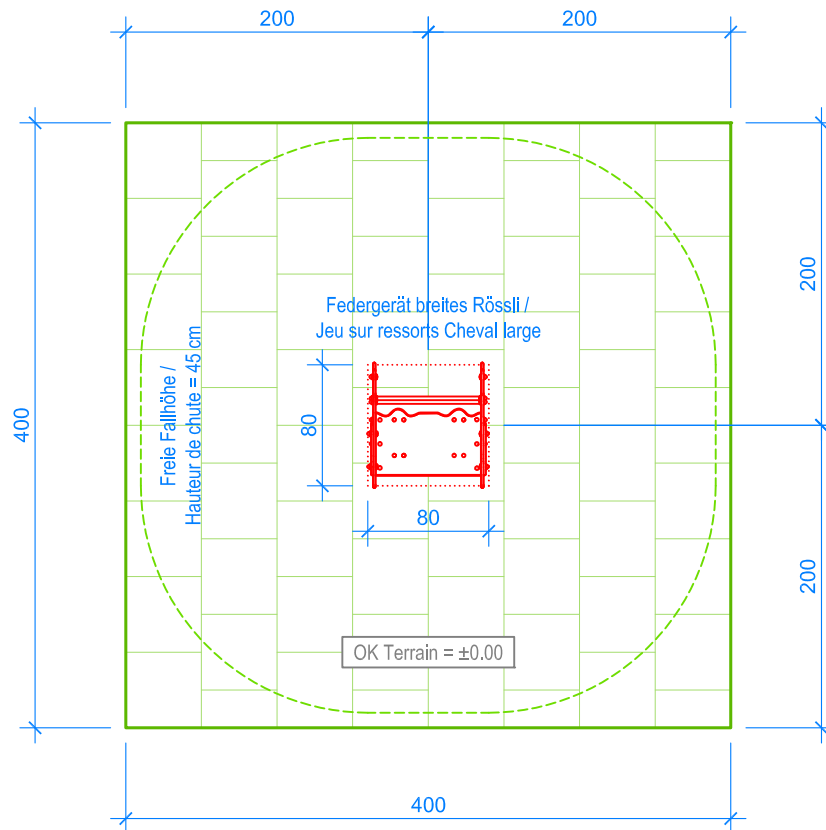
GRUNDRISS / PLAN 1:50
