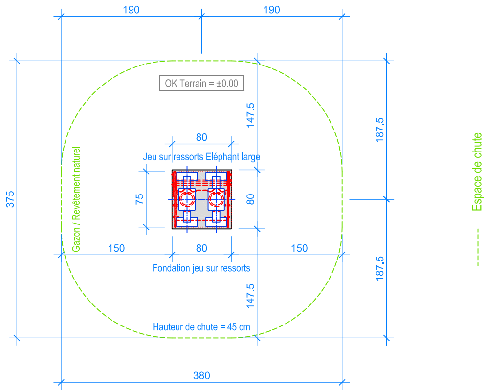
PLAN 1:50
