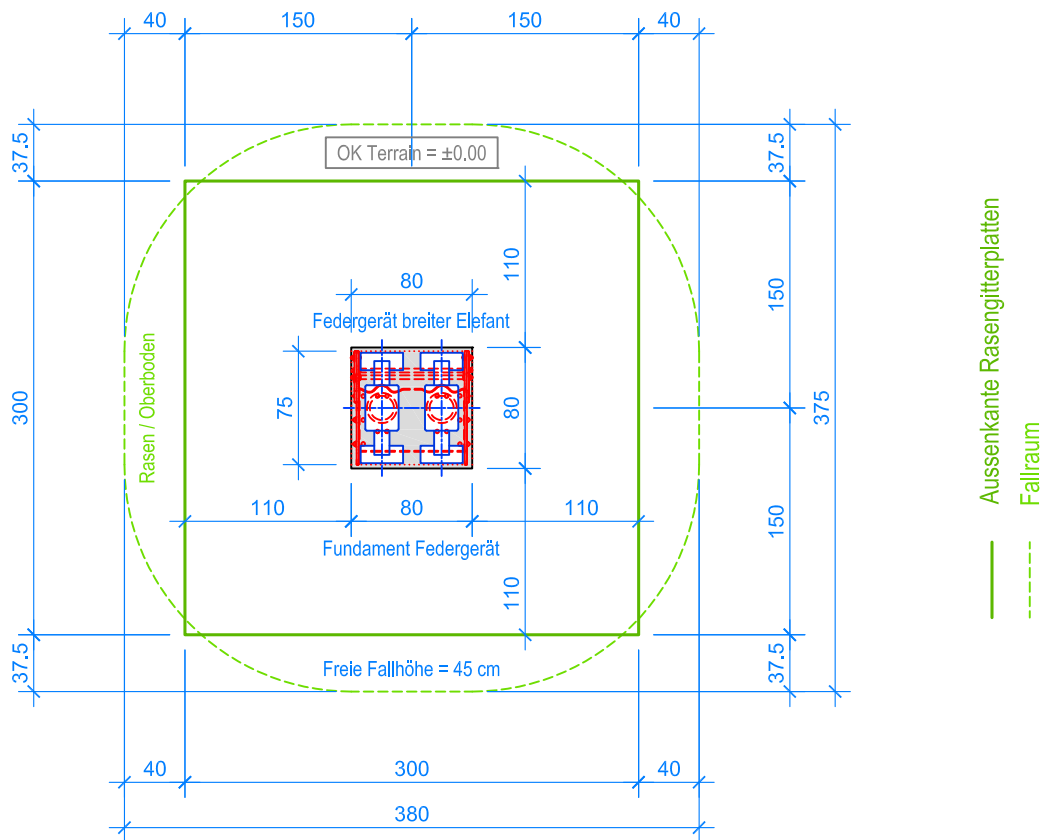
GRUNDRISS 1:50
