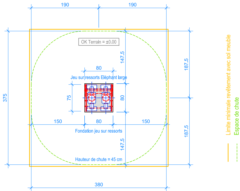
PLAN 1:50
