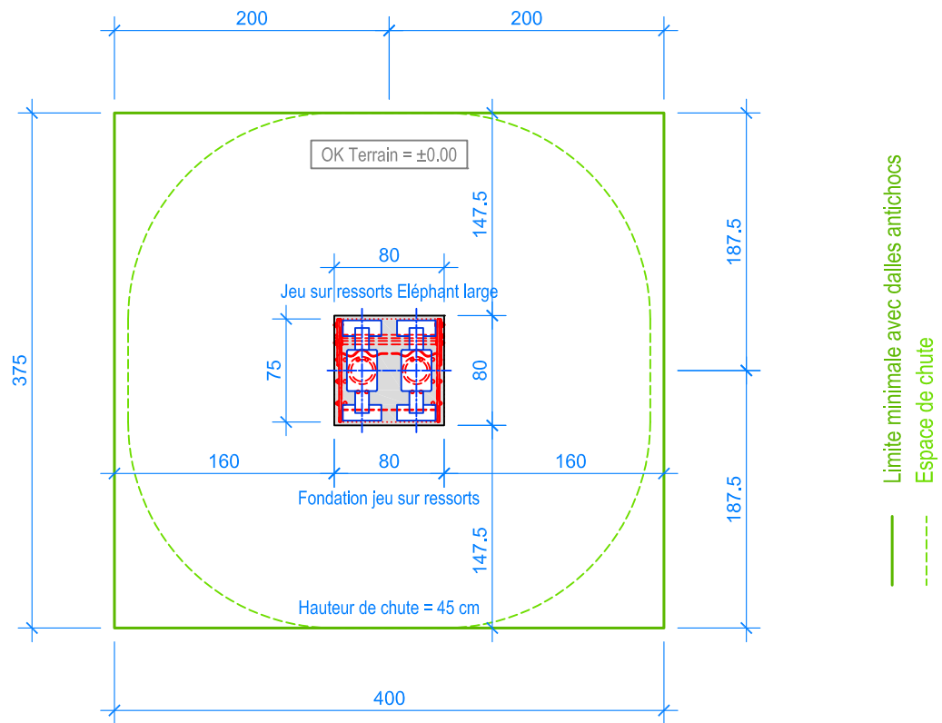
PLAN 1:50
