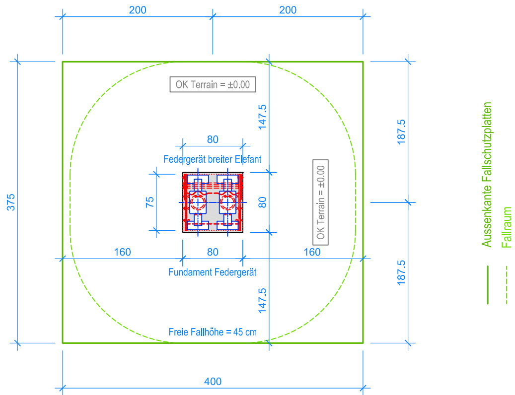
GRUNDRISS 1:50
