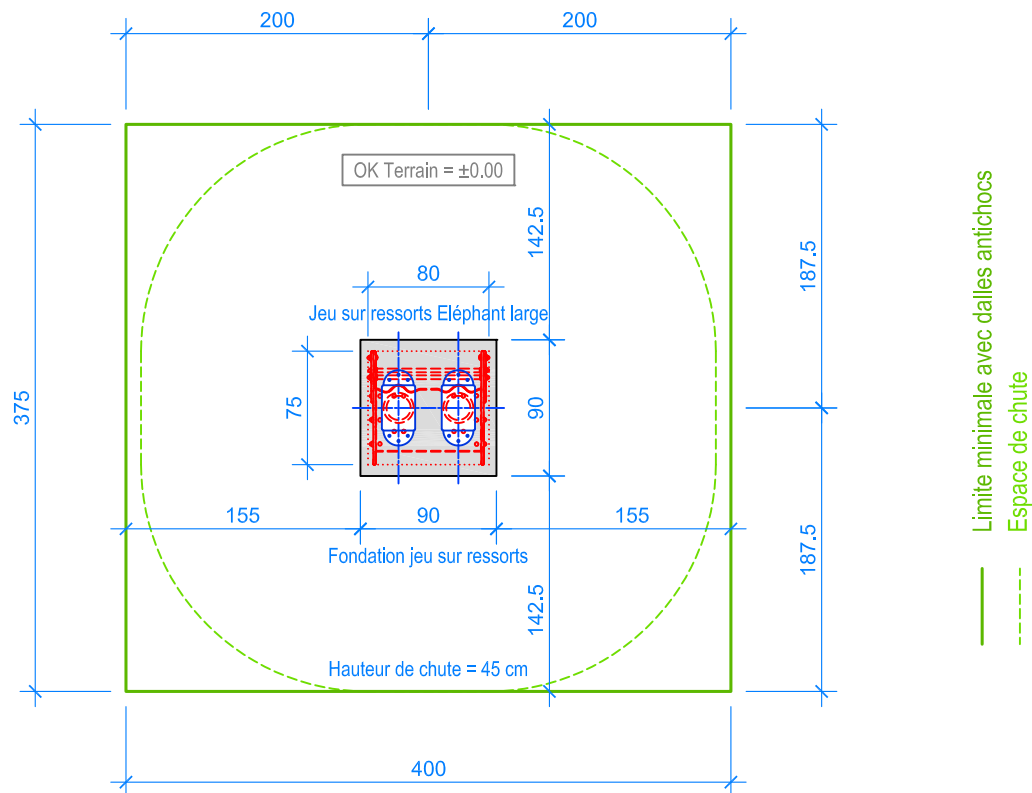
PLAN 1:50
