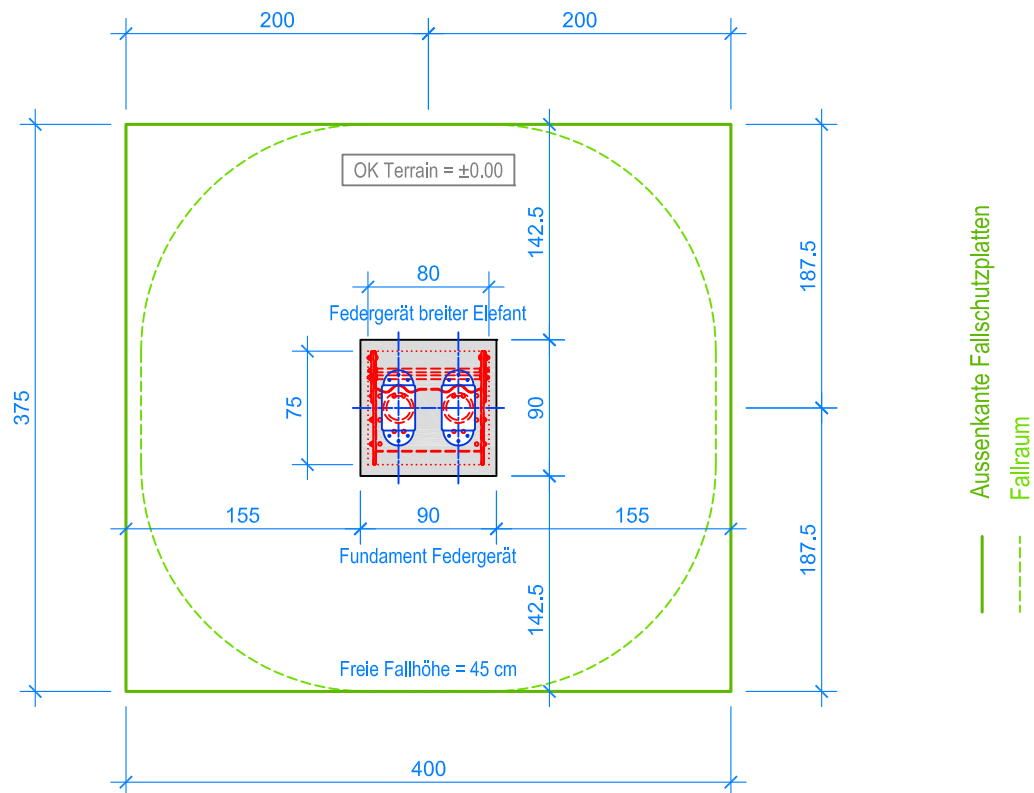
GRUNDRISS 1:50
