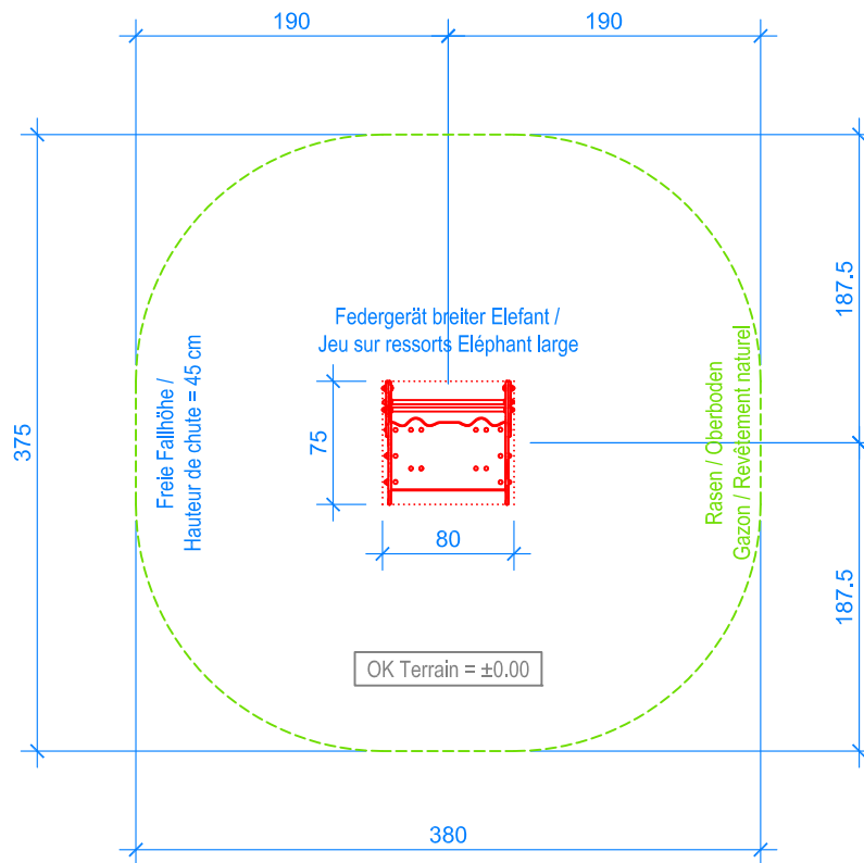
GRUNDRISS / PLAN 1:50
