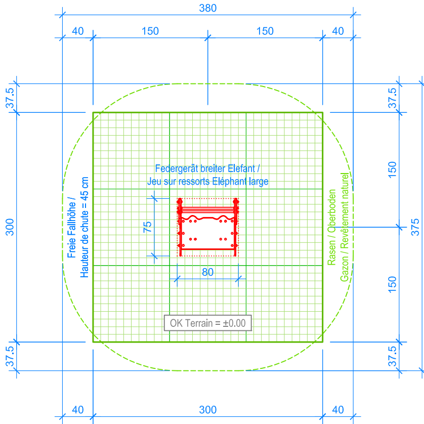
GRUNDRISS / PLAN 1:50
