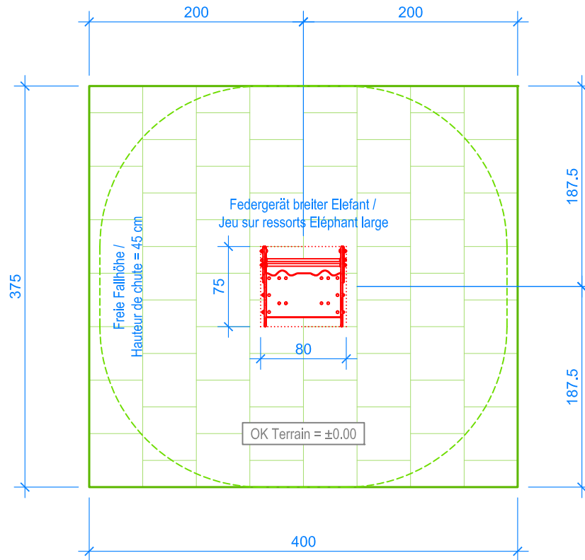
GRUNDRISS / PLAN 1:50
