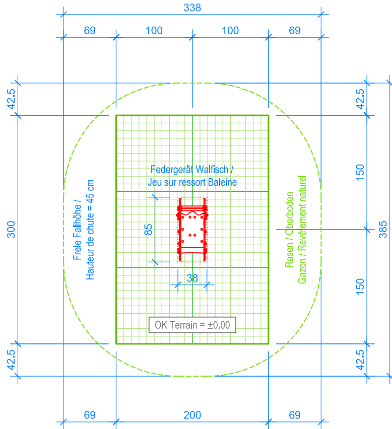
GRUNDRISS / PLAN 1:50
