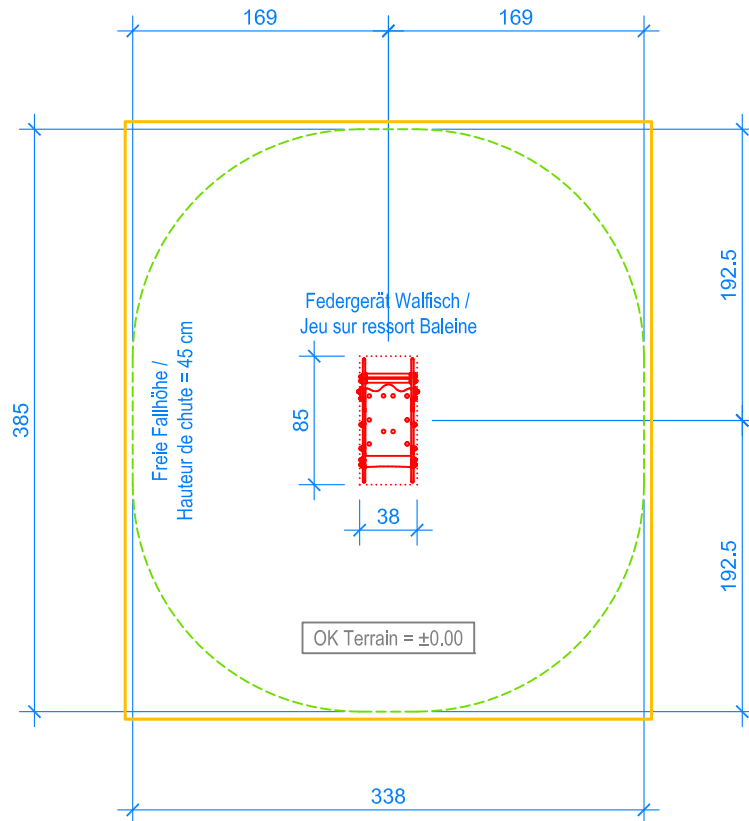
GRUNDRISS / PLAN 1:50
