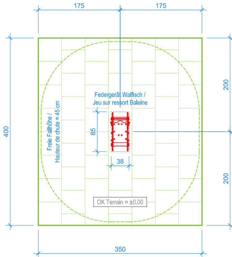
GRUNDRISS / PLAN 1:50
