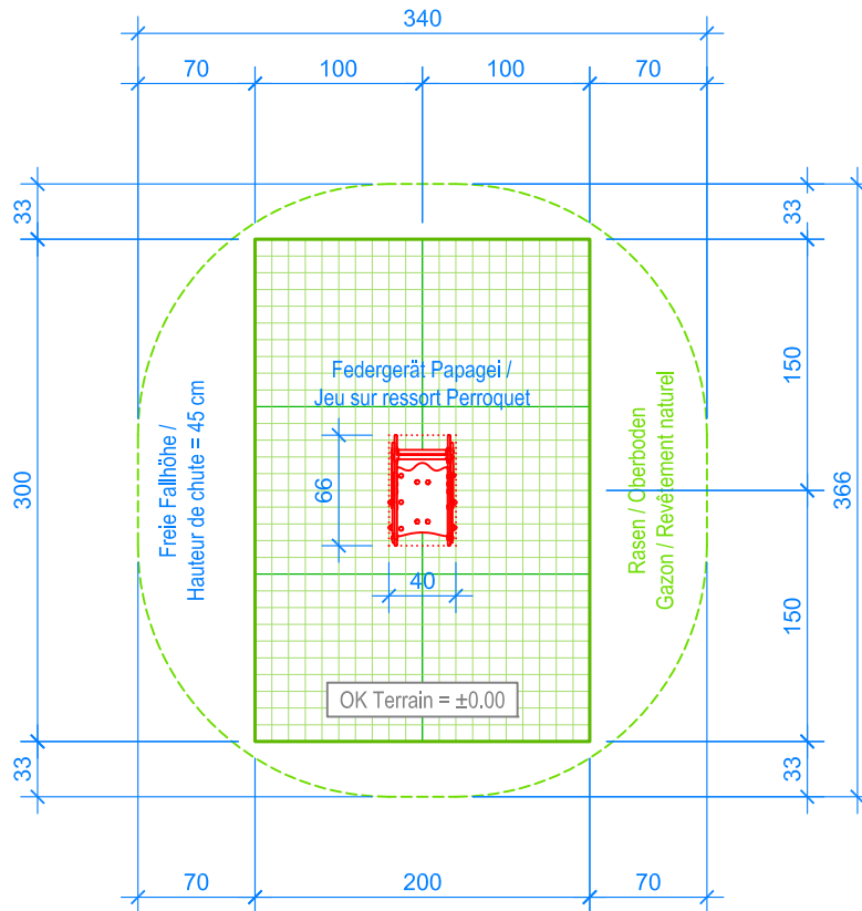
GRUNDRISS / PLAN 1:50
