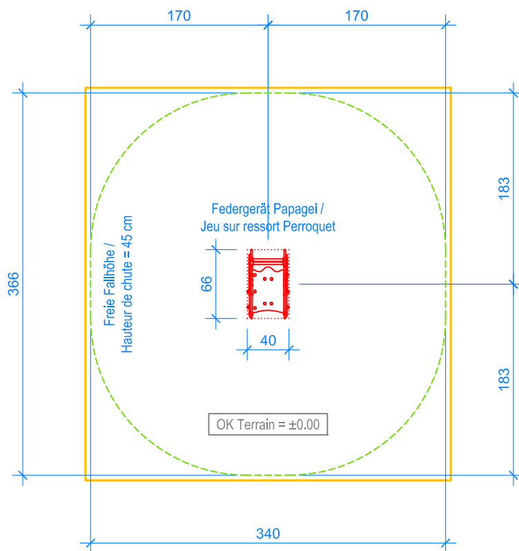
GRUNDRISS / PLAN 1:50
