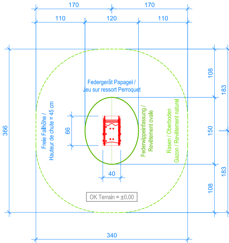
GRUNDRISS / PLAN 1:50
