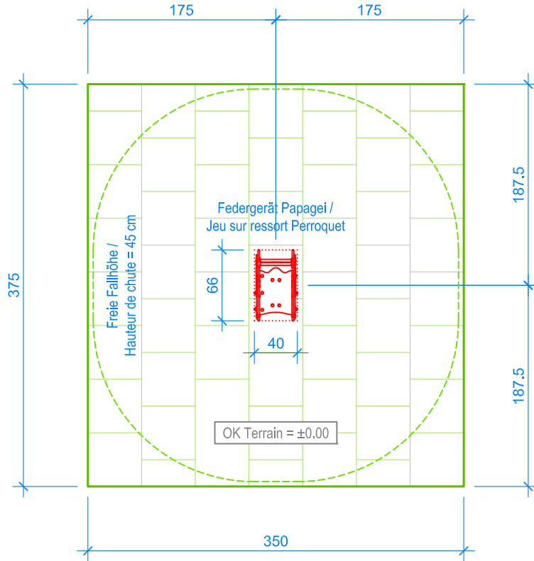
GRUNDRISS / PLAN 1:50
