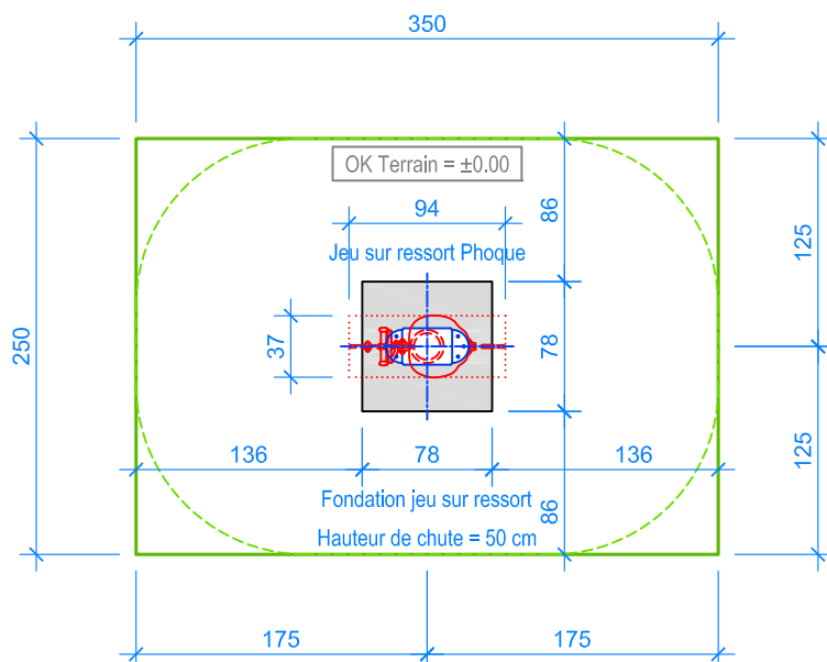
PLAN 1:50
