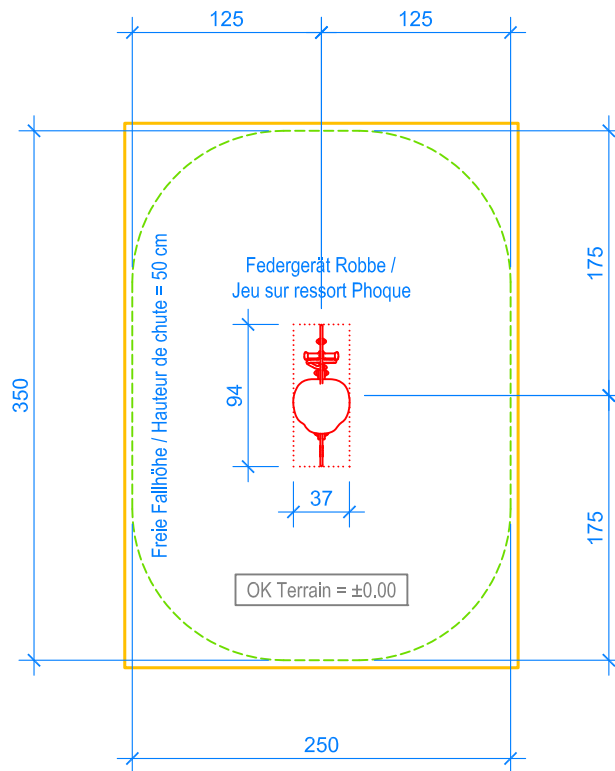
GRUNDRISS / PLAN 1:50
