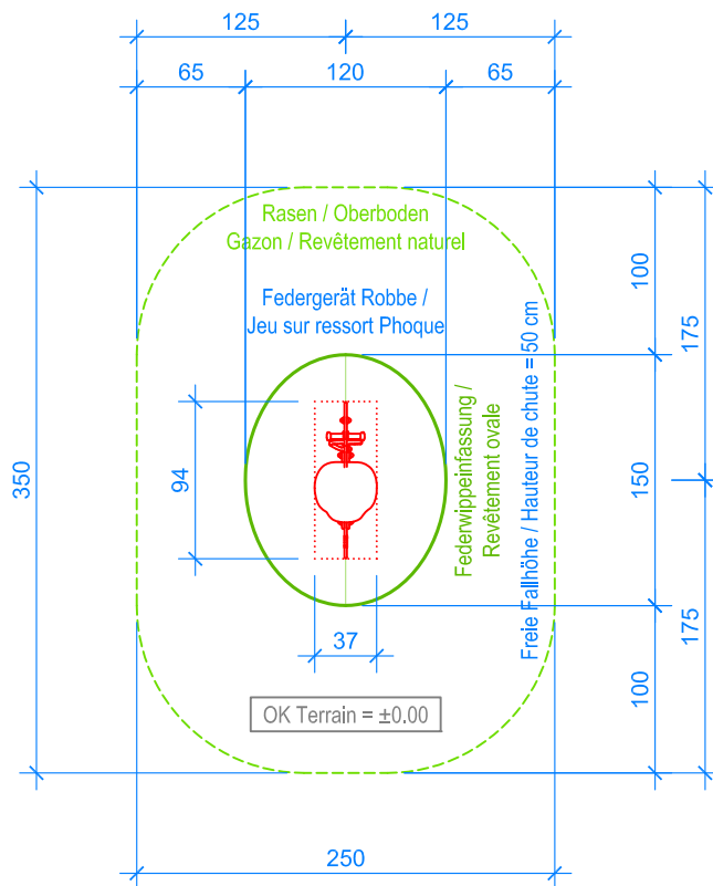
GRUNDRISS / PLAN 1:50
