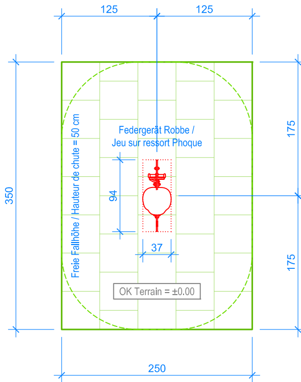
GRUNDRISS / PLAN 1:50
