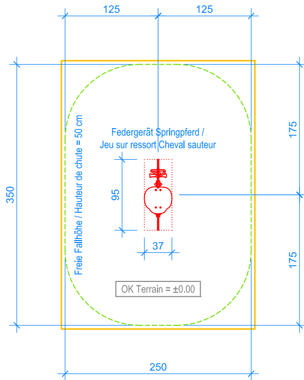
GRUNDRISS / PLAN 1:50
