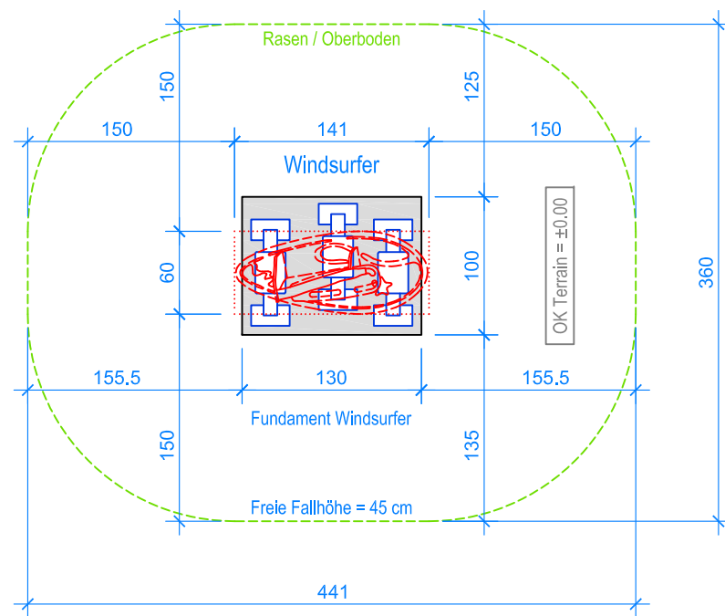
GRUNDRISS 1:50
