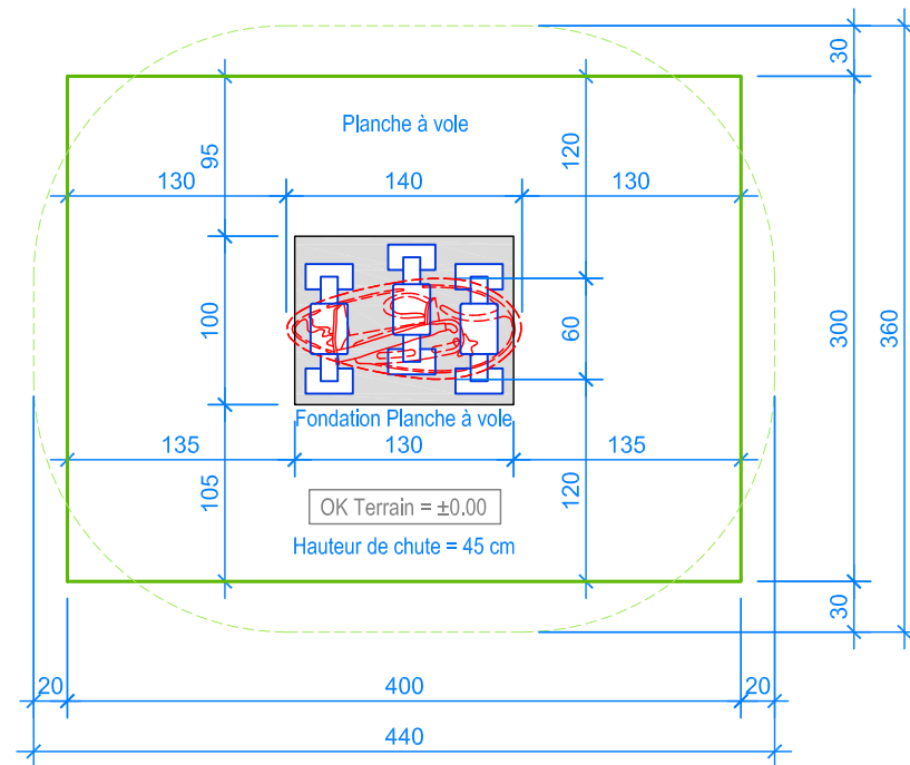
PLAN 1:50
