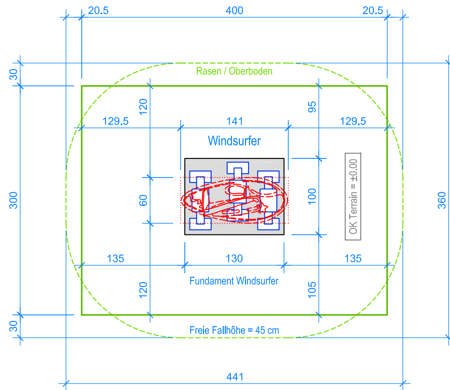
GRUNDRISS 1:50
