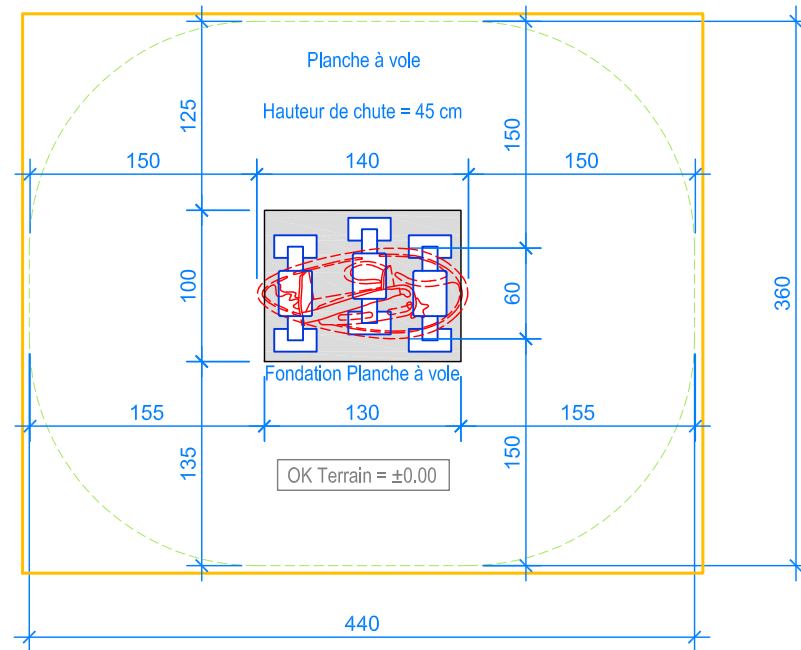
PLAN 1:50
