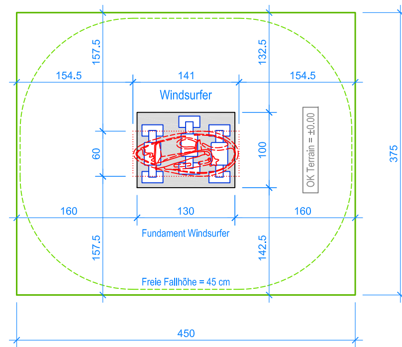
GRUNDRISS 1:50
