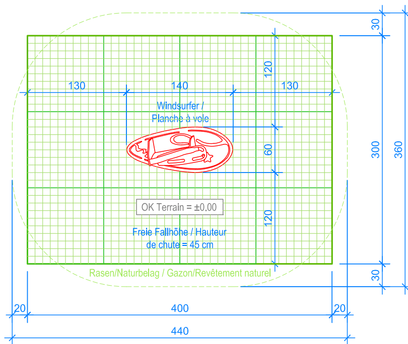
GRUNDRISS / PLAN 1:50
