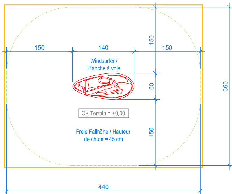
GRUNDRISS / PLAN 1:50
