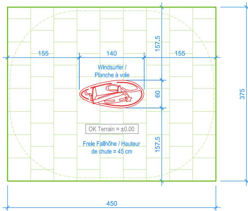
GRUNDRISS / PLAN 1:50
