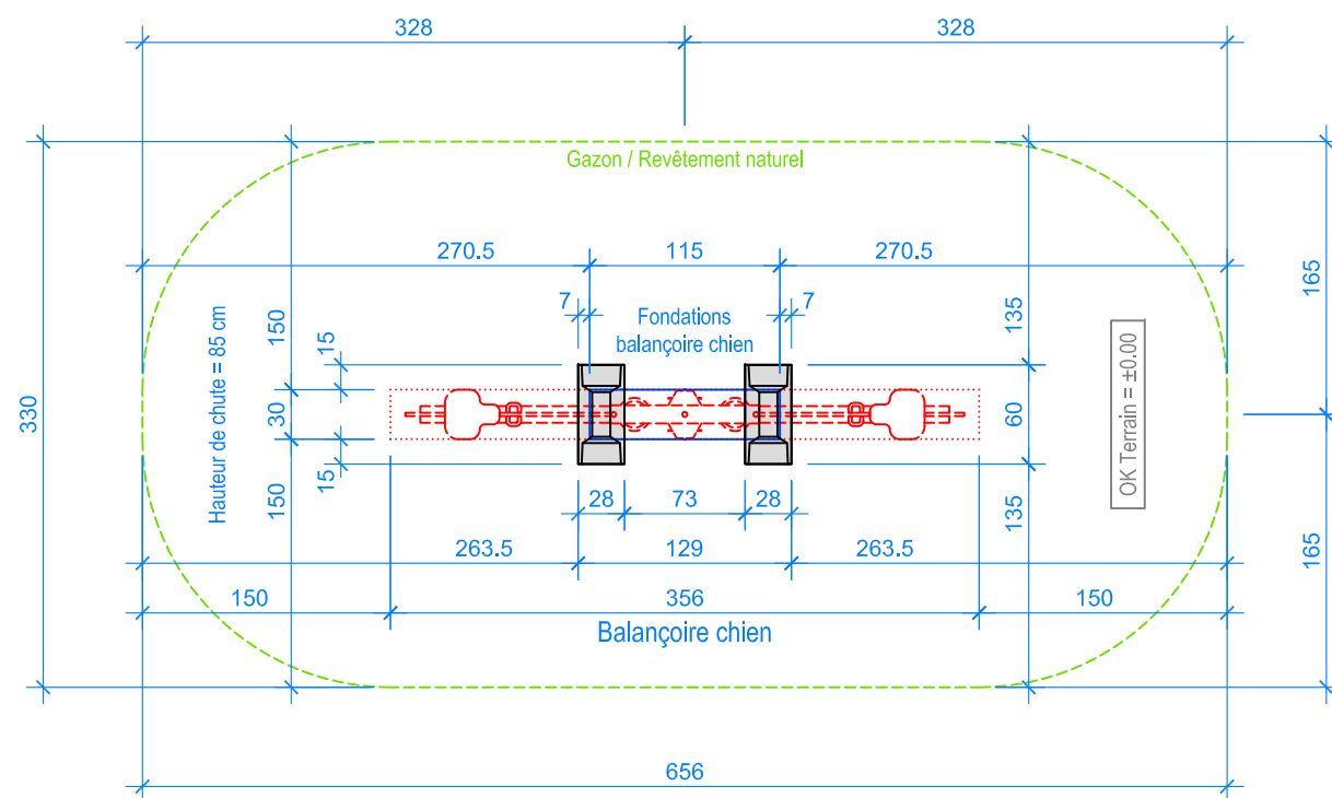
PLAN 1:50
