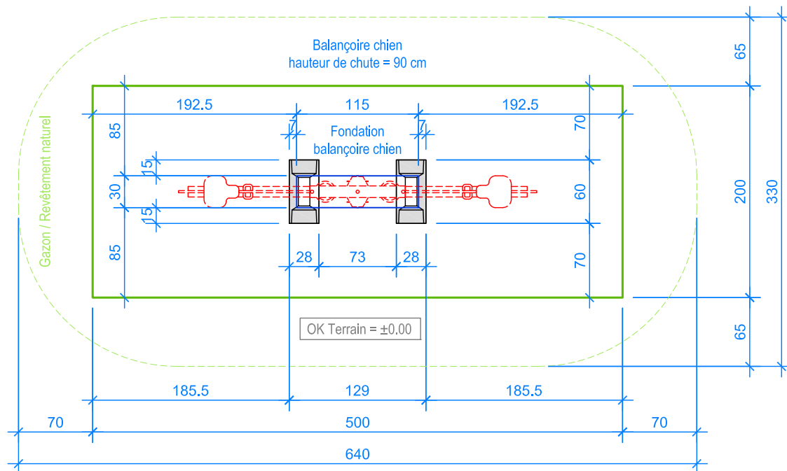
PLAN 1:50
