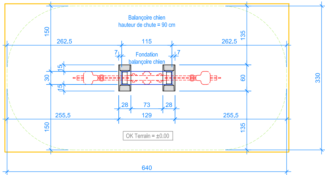
PLAN 1:50
