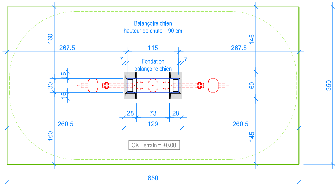
PLAN 1:50
