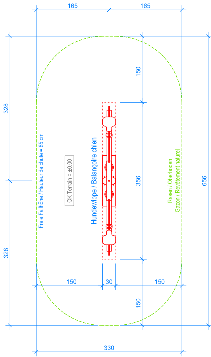
GRUNDRISS / PLAN 1:50
