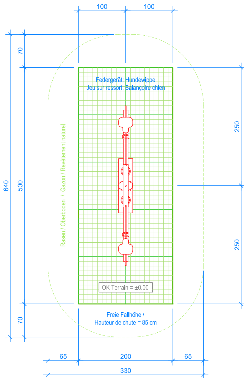
GRUNDRISS / PLAN 1:50
