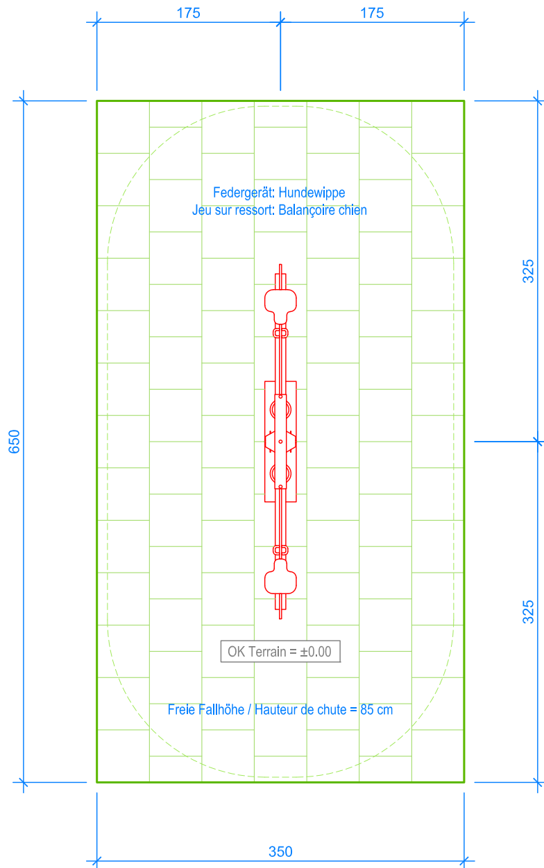
GRUNDRISS / PLAN 1:50
