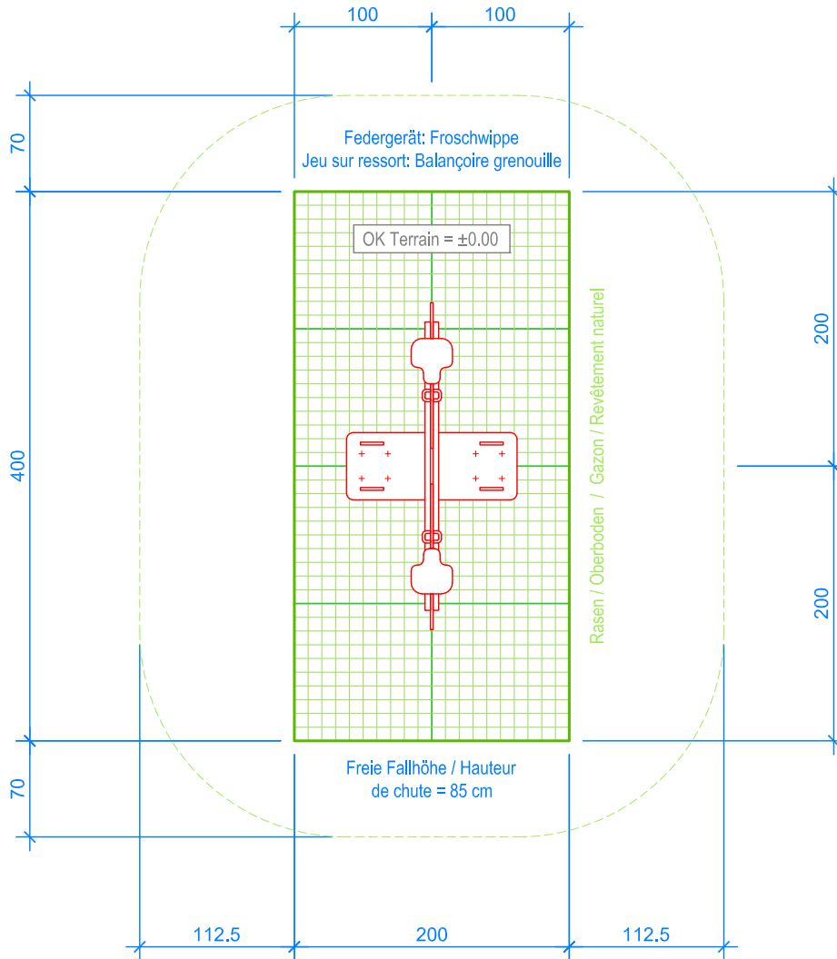
GRUNDRISS / PLAN 1:50
