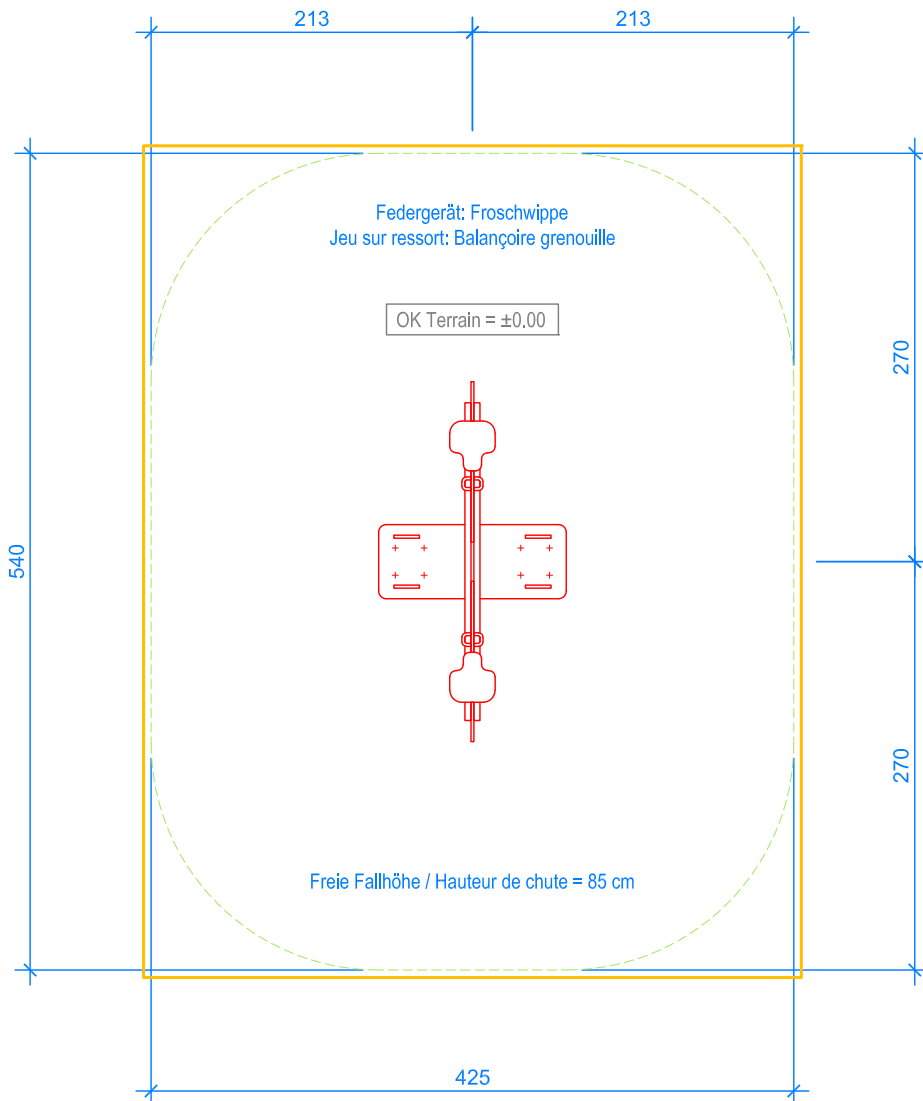
GRUNDRISS / PLAN 1:50
